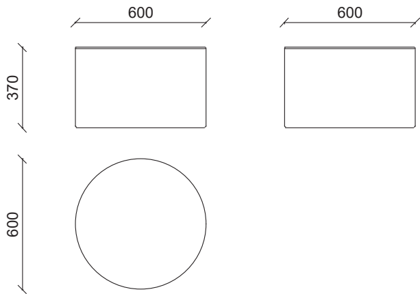
Ø 600 X H 370 MM
