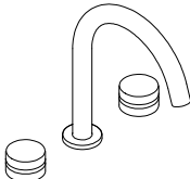
3-hole washbasin set, swivel spout D 176 H 252 mm Batteria lavabo 3 fori bocca girevole P 176 H 252 mm
